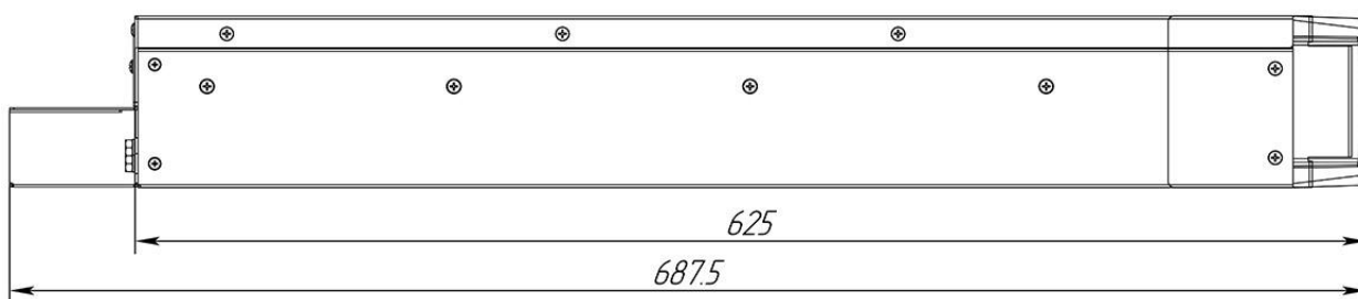
Вид сбоку
