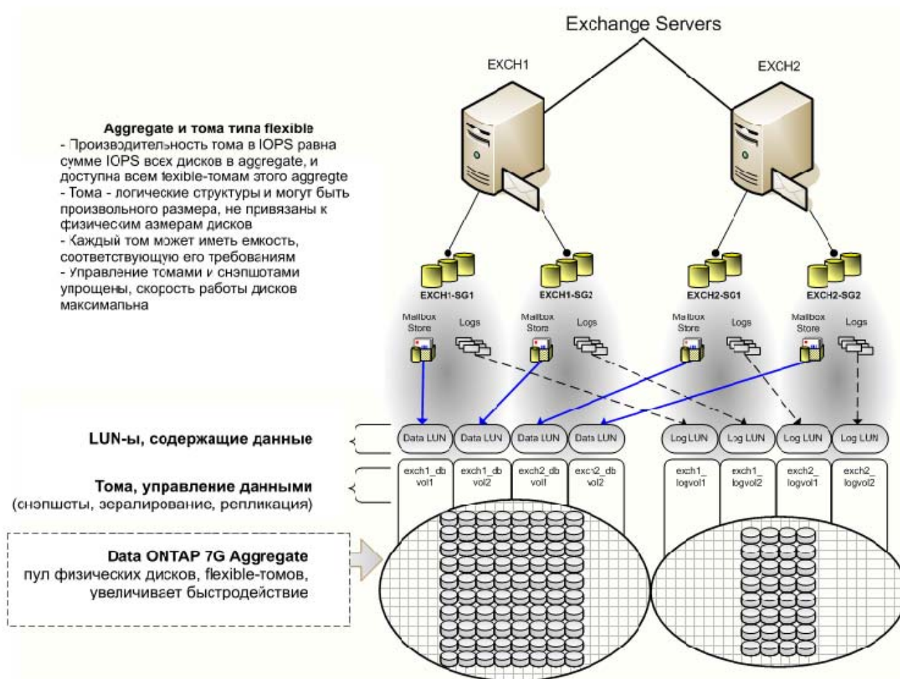
Рис. 2) Использование Data ONTAP 7G и flexible volumes.
